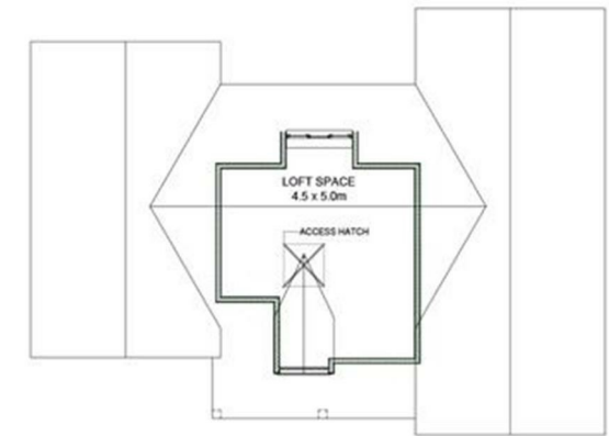
LOFT PLAN
